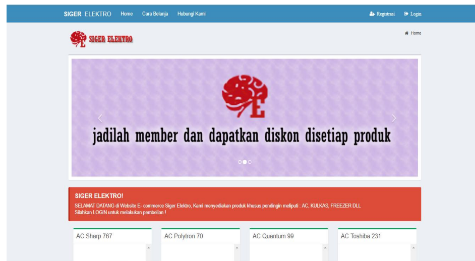
Gambar 4.40 Halaman Utama
