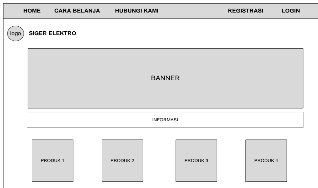
Gambar 4.8 Halaman utama
