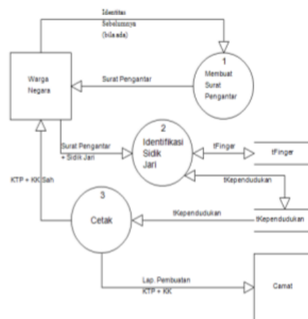
Gambar 4. Data flow diagram pengembangan sistem
