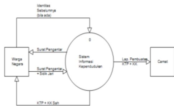
Gambar 3. Context diagram pengembangan sistem
