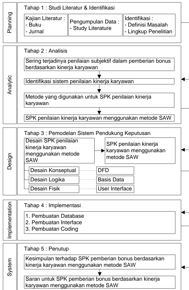
Gambar 3.1 Tahapan Penelitian
