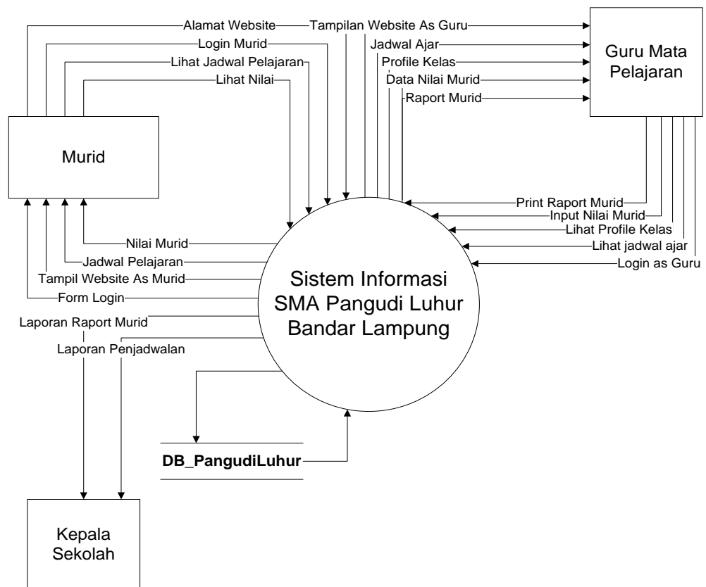
Gambar 4.3 Context Diagram Sistem Yang Diusulkan
