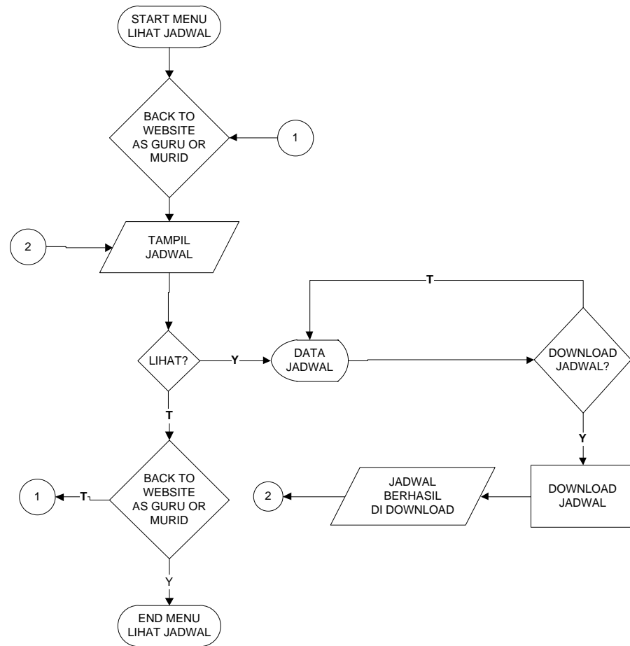
.Gambar 4.35 Flowchart Program Menu Lihat Jadwal
