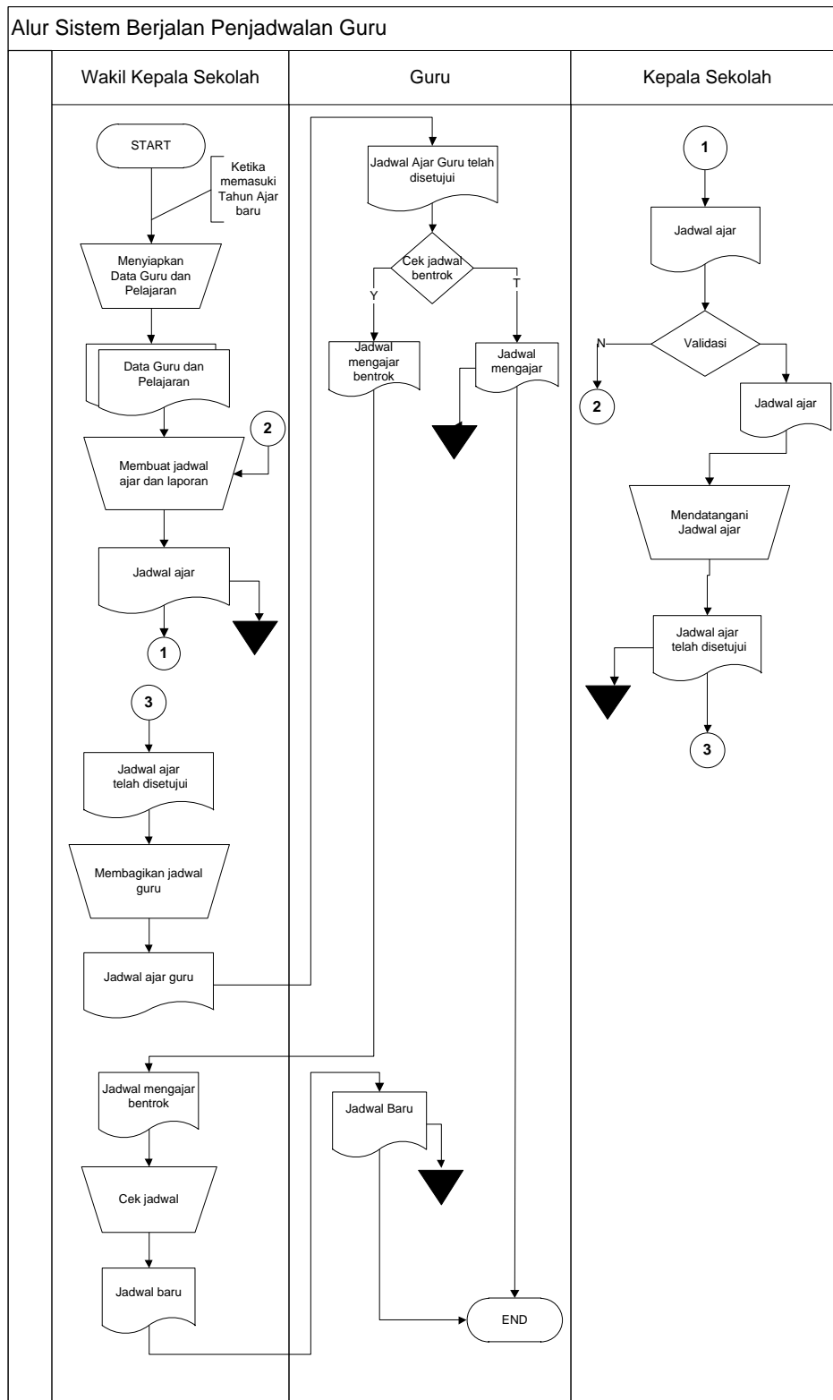
Gambar 4.1 Bagan Alir Dokumen Penjadwalan Guru SMA Pangudi Luhur Bandar Lampung
