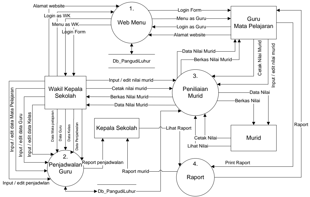
Gambar 4.4 DFD Level 0 sistem yang diusulkan
