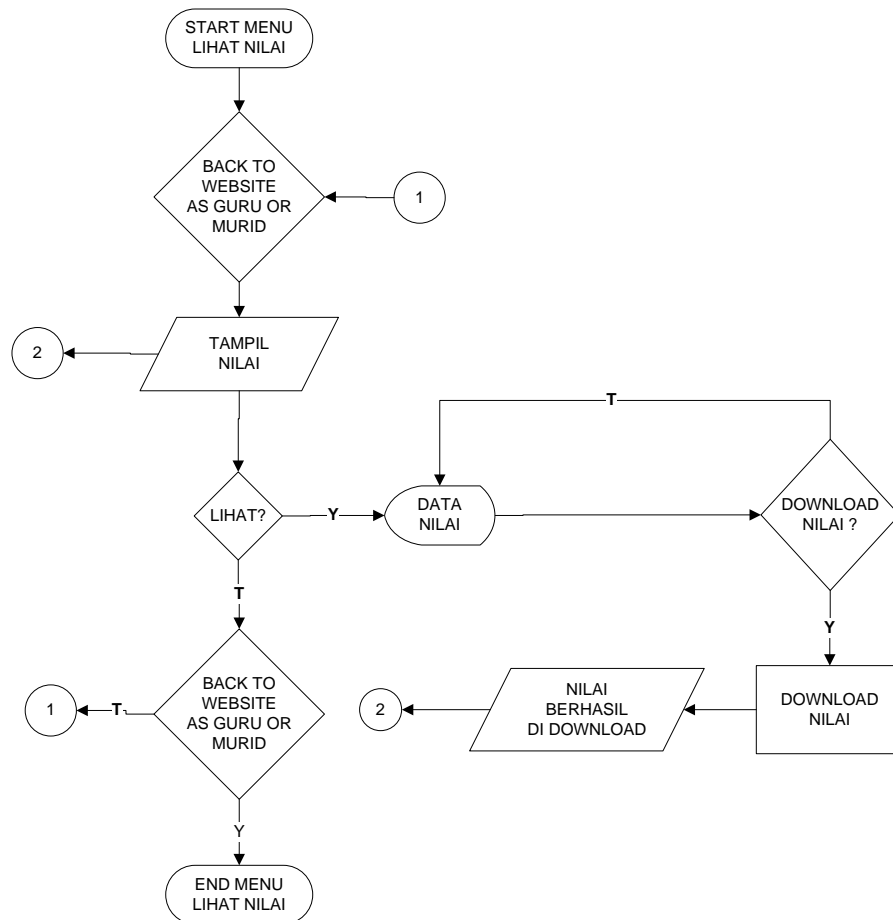
Gambar 4.36 Flowchart program menu lihat nilai.
