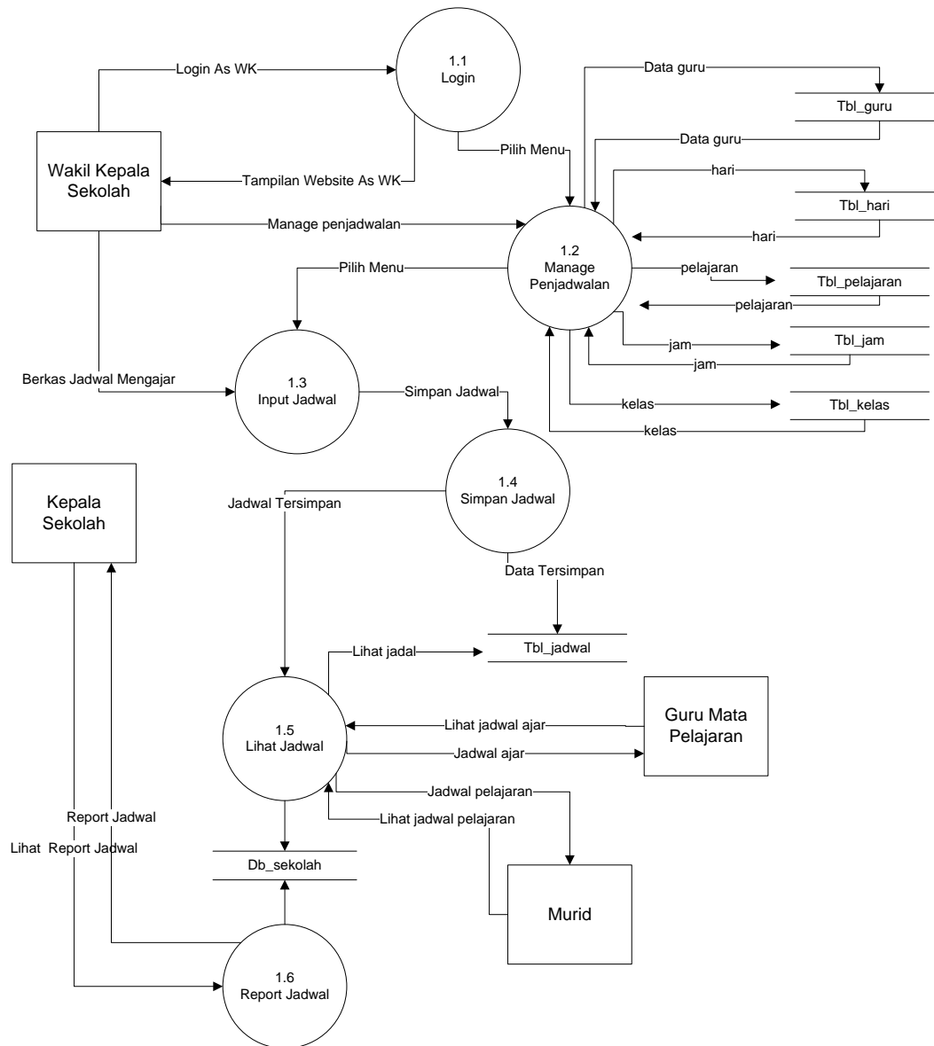
Gambar 4.5 DFD Level 1 Proses 1 Sub Sistem Penjadwalan.
