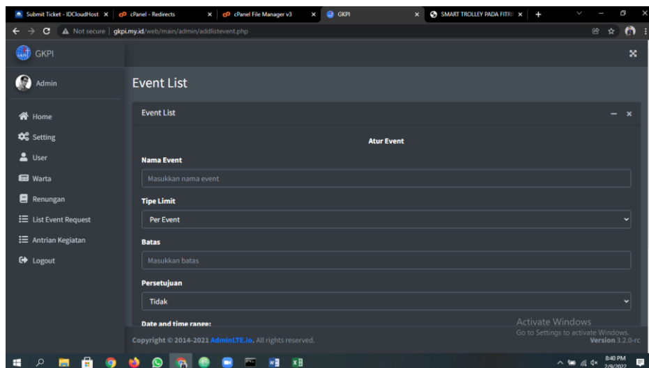
Gambar 4.3 Tampilan Antarmuka Tambah Event .
