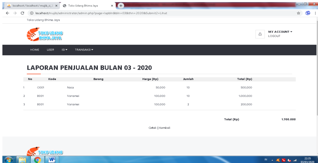
Gambar 4.24 Halaman Laporan Perbulan
