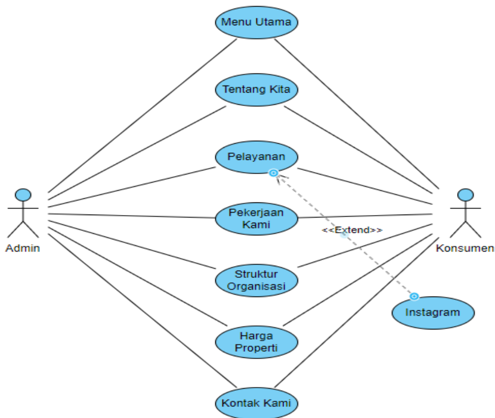
Gambar 1.1 Use Case Diagram Web Profile Perusahaan.
