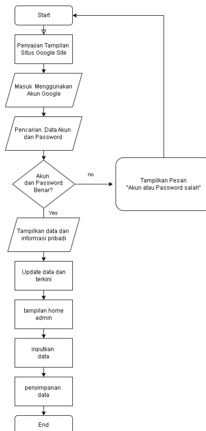
Gambar 1.1 Pembuatan Flowchart Website
