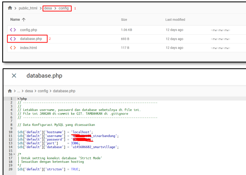
Gambar 2.8 Tampilan Konfigurasi Database
