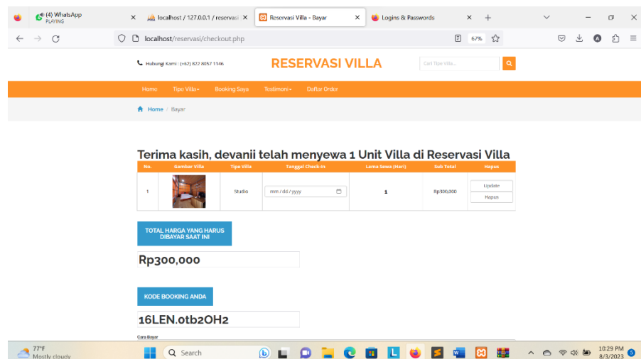
Gambar 4.6 Tampilan Pembayaran
