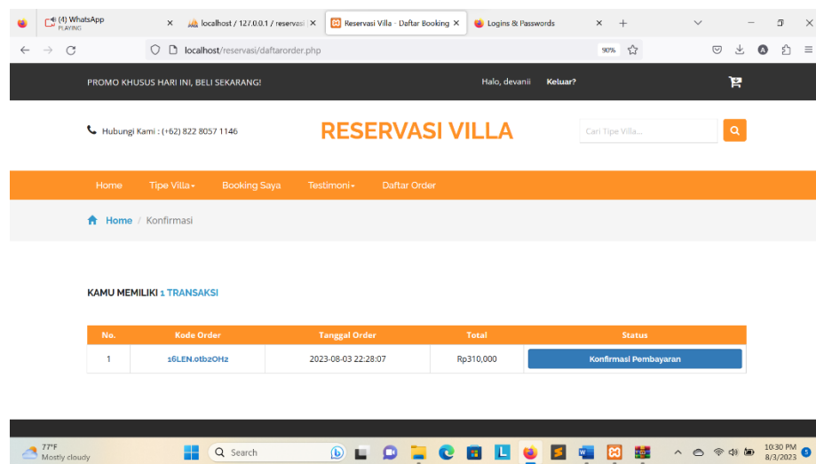
Gambar 4.7 Tampilan Konfirmasi
