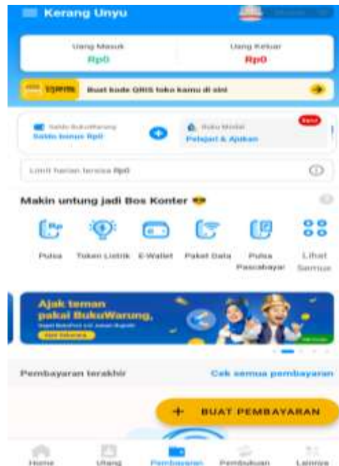
Gambar 2.9 fitur pembayaran
