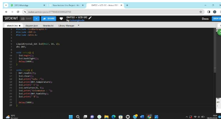
Gambar 2. 4 source code pada wokwi
