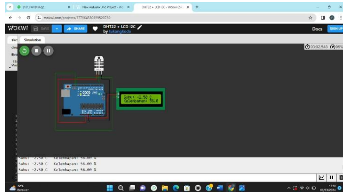
Gambar 2. 3 simulasi rangkaian alat pada wokwi
