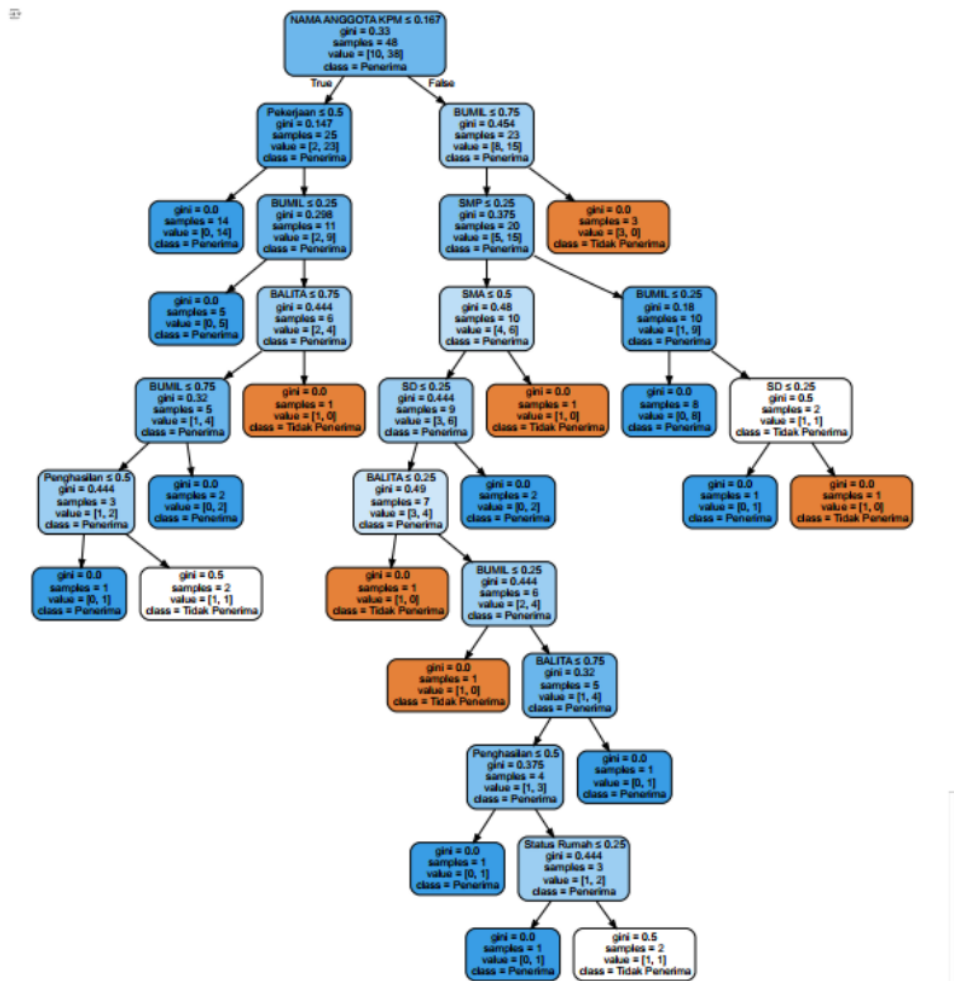
Gambar 3. 5 Pohon CART
