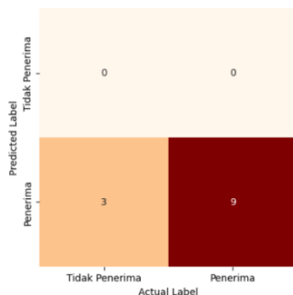
Gambar 3. 3 Visualisasi Data Heatmap
