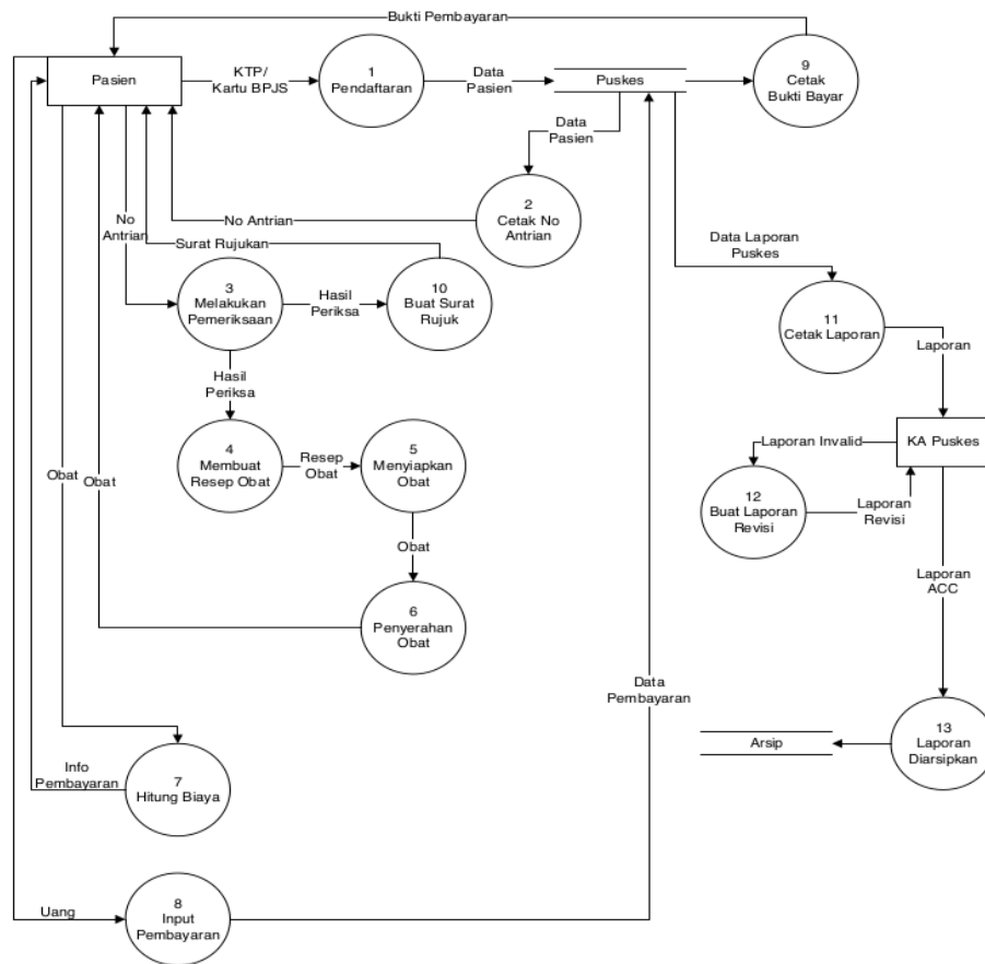
Gambar 5. DFD level 0 Pengolahan Data Puskesmas.
