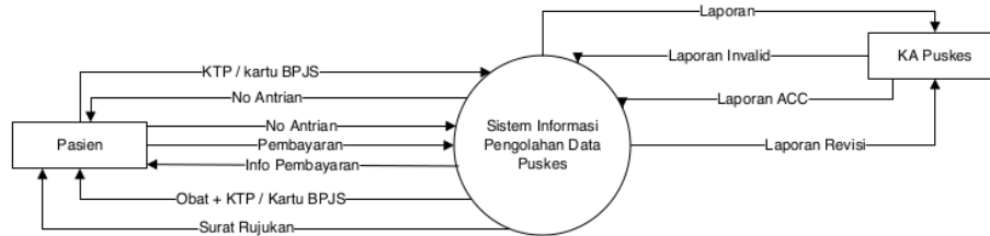
Gambar 4. Context diagram Sistem Diusulkan
