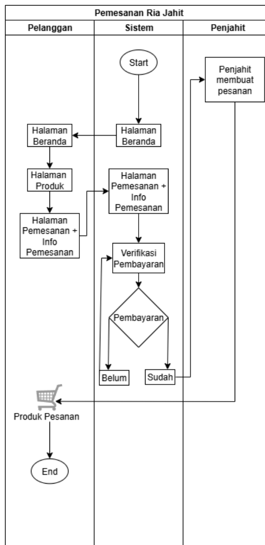
Gambar 2.5 Sistem Di Usulkan Web Ria Jahit
