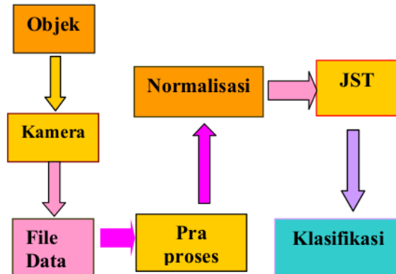
GAMBAR 3.1. ARSITEKTUR SISTEM
