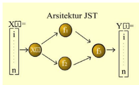
Gambar 3.2 Arsitektur jaringan
