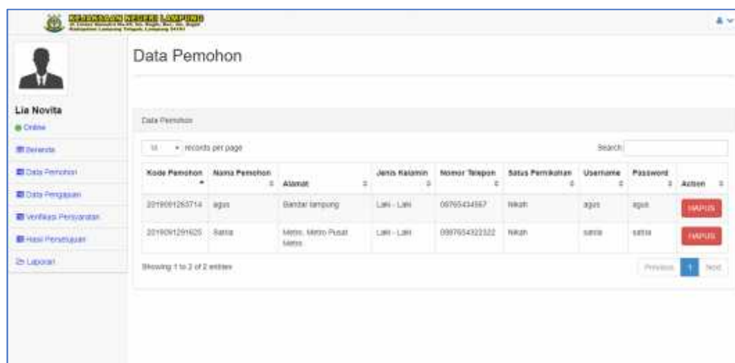
Gambar 4.3. Implementasi Antar Muka Data Pelanggan
