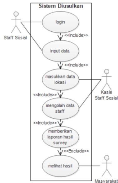
Gambar 3. Use Case Diagram Sistem Diusulkan
