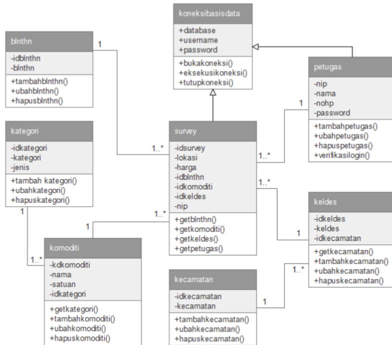
Gambar 10. Perancangan Clas Diagram Sistem diusulkan
