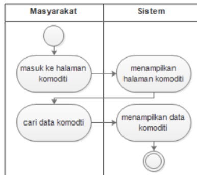
Gambar 9. Perancangan Activity Diagram Lihat Hasil
