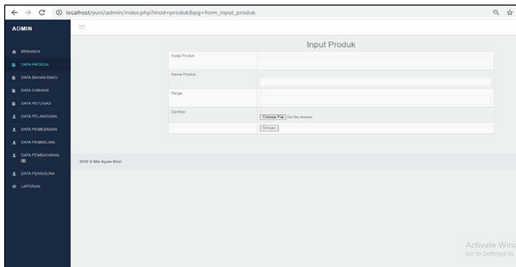
Gambar 4.4 Tambah Produk
