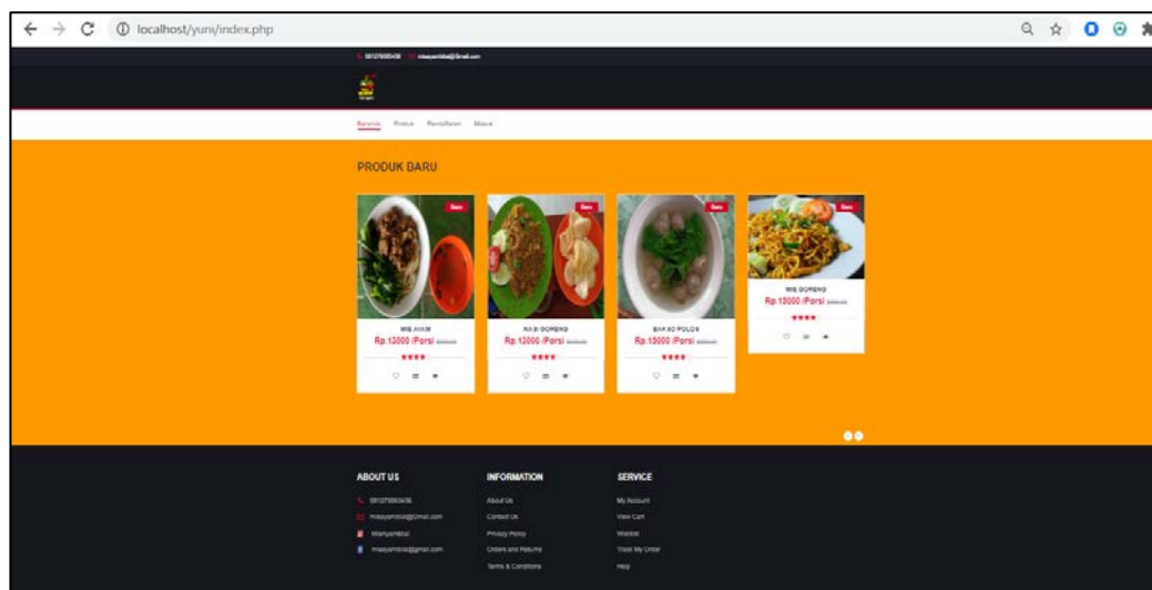
Gambar 4.1 Menu Utama
