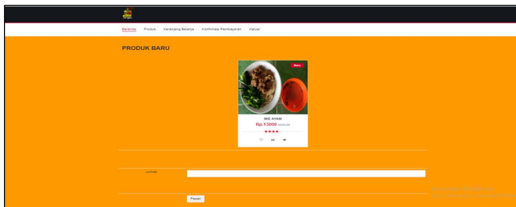
Gambar 4.22 Menu Produk
