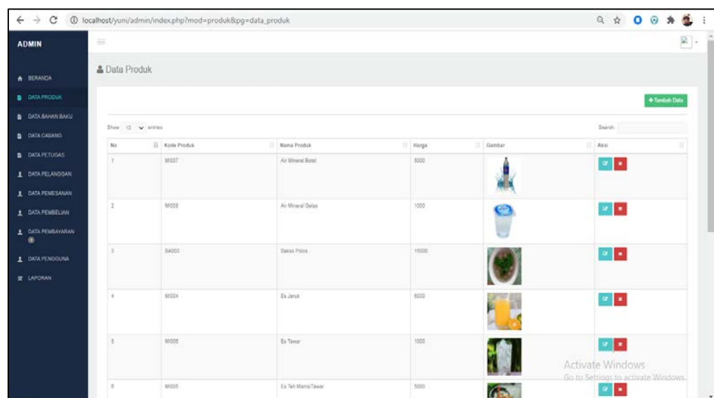
Gambar 4.5 Menu Produk
