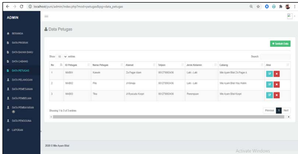
Gambar 4.10 Data Petugas
