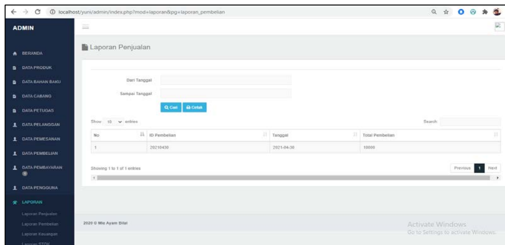
Gambar 4.18 Laporan Pembelian
