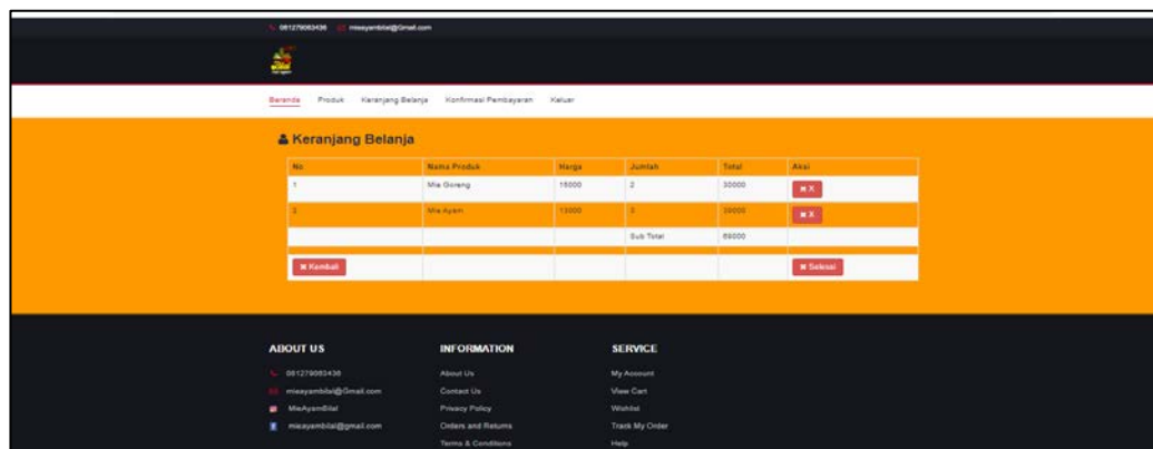
Gambar 4.23 Keranjang Belanja
