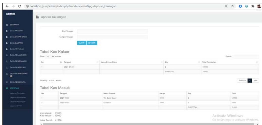
Gambar 4.19 Laporan Keuangan
