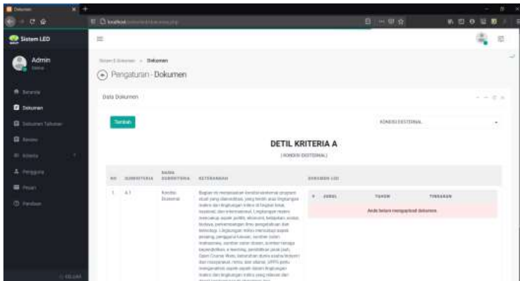
Gambar 4.4 Halaman Dokumen
