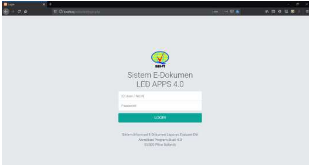
Gambar 4.1 Halaman Login
