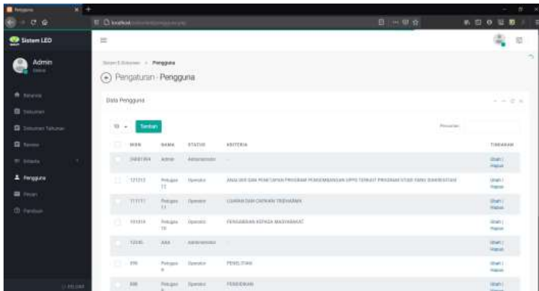
Gambar 4.10 Halaman Pengguna
