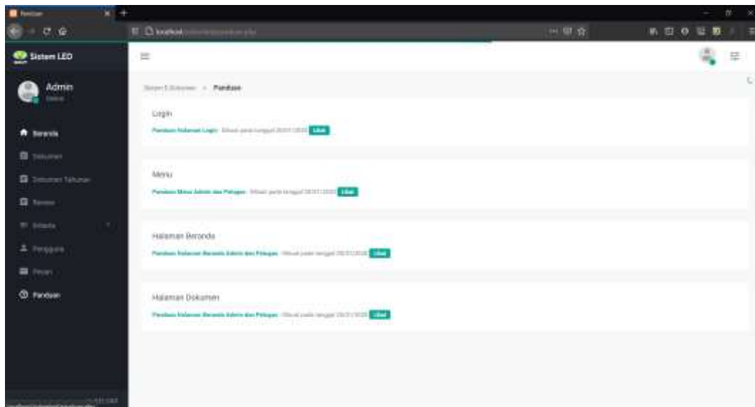
Gambar 4.12 Halaman Panduan
