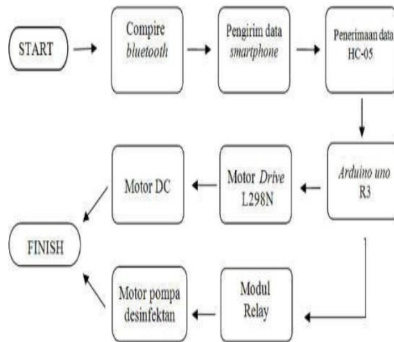
Gambar 2.2 Blok Diagram Pengembangan Sistem
