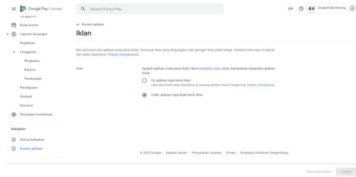
Gambar 4. 35 setelan periklanan
