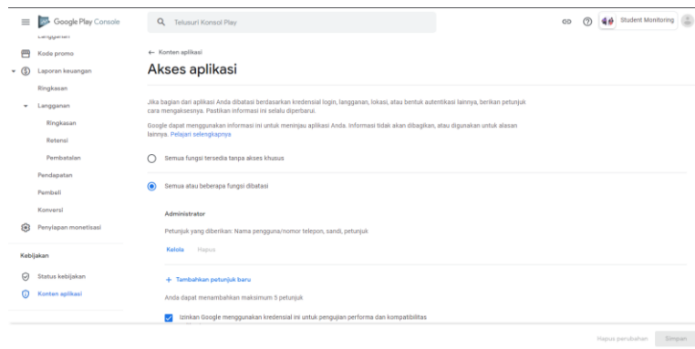
Gambar 4. 36 mengisi kuisioner
