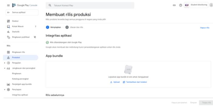
Gambar 4. 41 upload aplikasi
