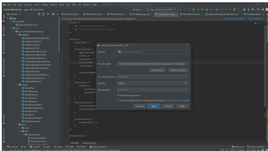
Gambar 4. 25 create keystore
