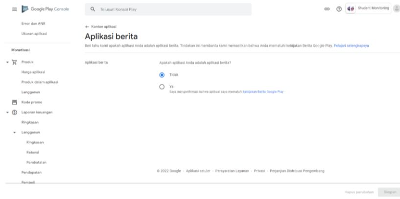
Gambar 4. 38 penargetan konten
