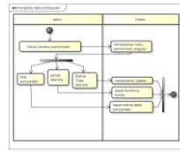
Gambar 4.10 Activity Diagram Mengelola Data Pembiayaan
