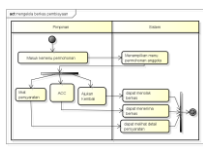
Gambar 4.14 Activity Diagram Mengelola Berkas Pembiayaan
