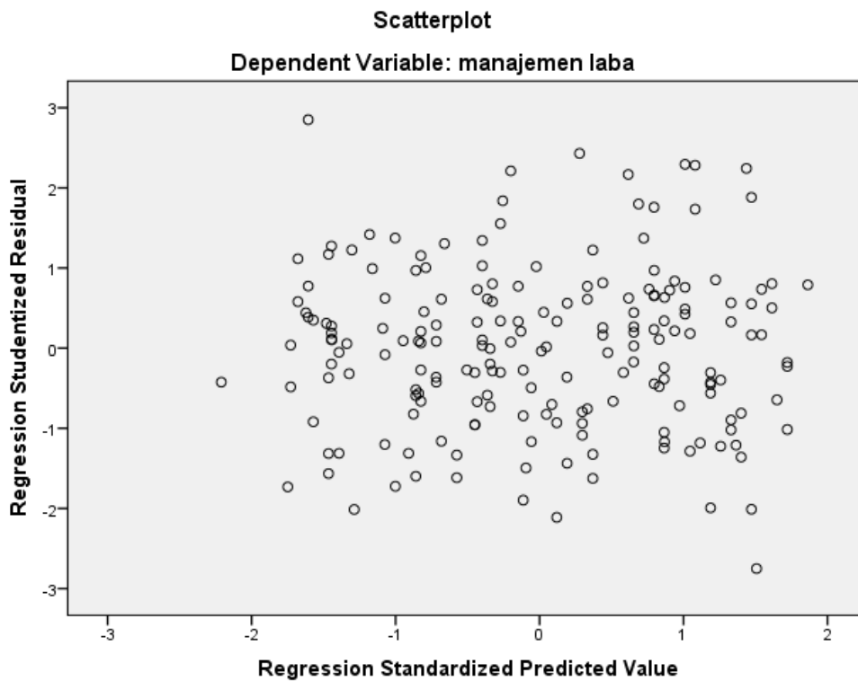
Gambar 4.1 Uji Heterokedositas
