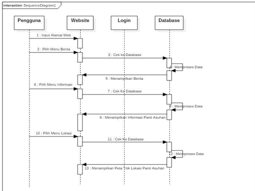
Gambar 4.7 Sequence Diagram Pengguna Sistem yang Diusulkan
