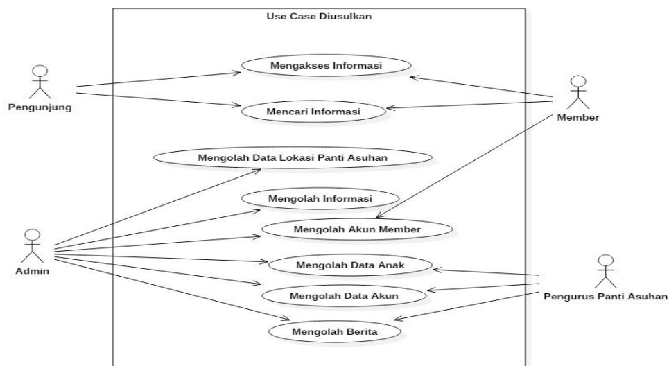
Gambar 4.2 Use Case Sistem yang diusulkan
