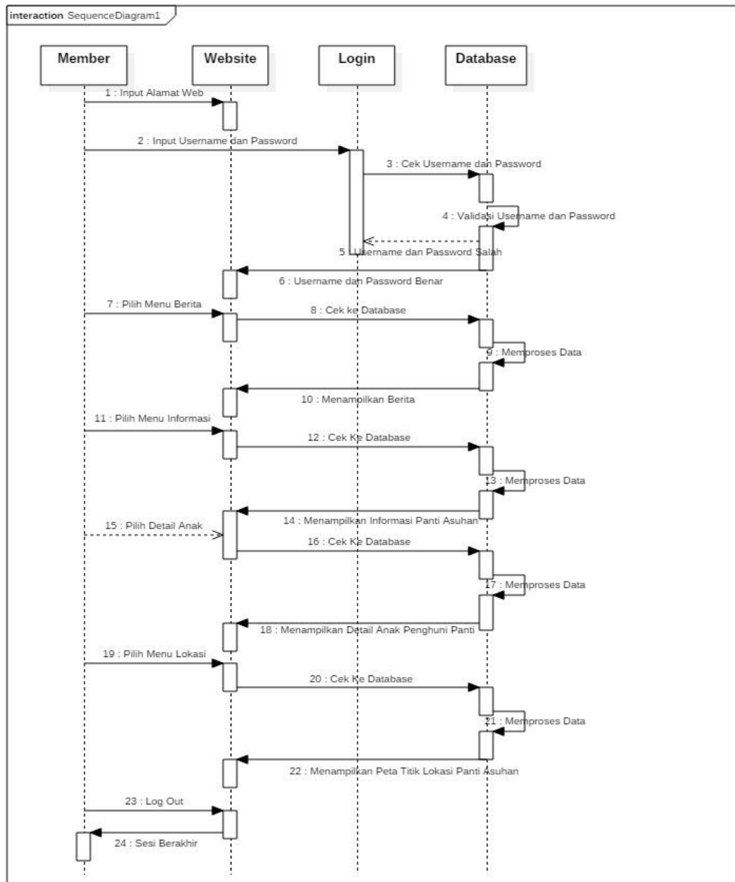
Gambar 4.6 Sequence Diagram Member Sistem yang Diusulkan
