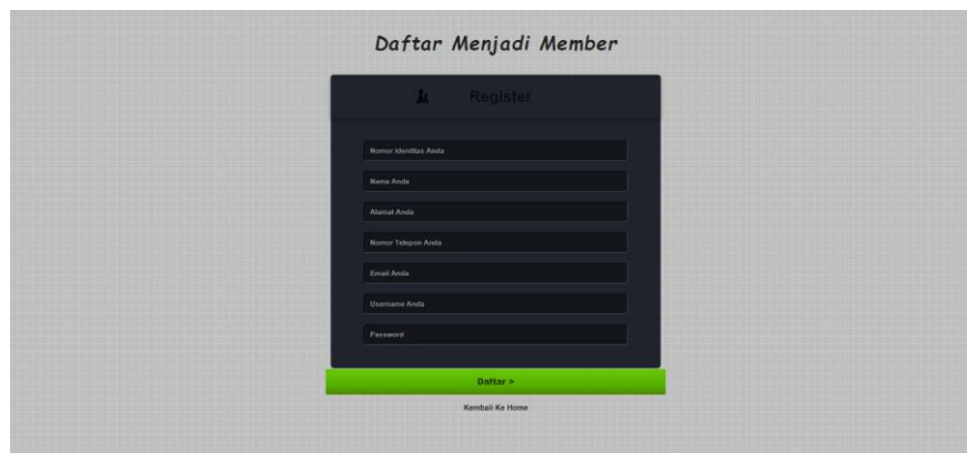
Gambar 4.50 Halaman Daftar
