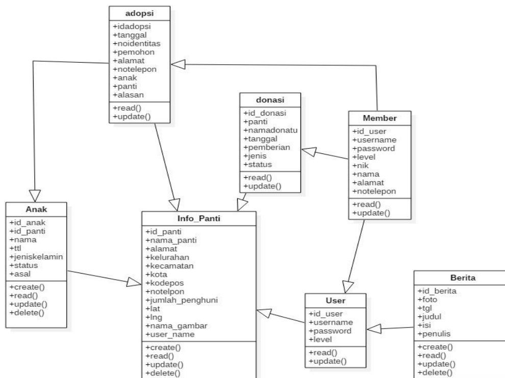
Gambar 4.8 Class Diagram Sistem diusulkan
