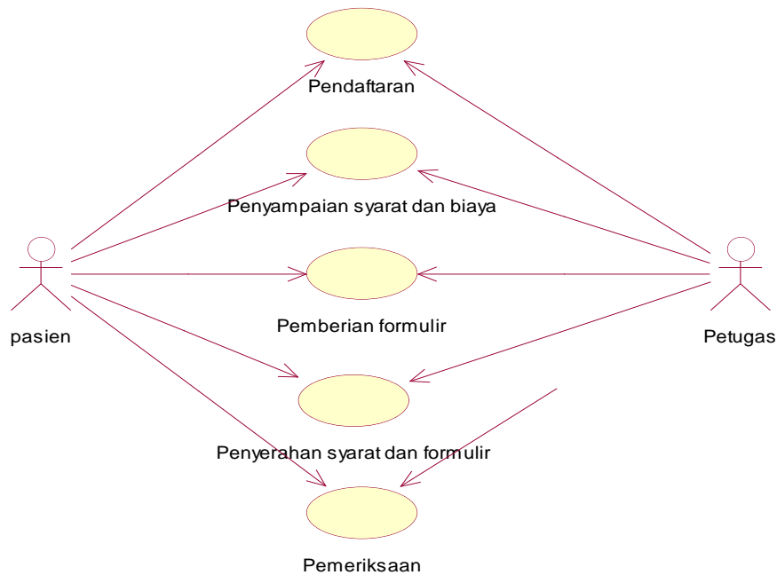
Gambar 4.1 Use Case Diagram sistem berjalan
