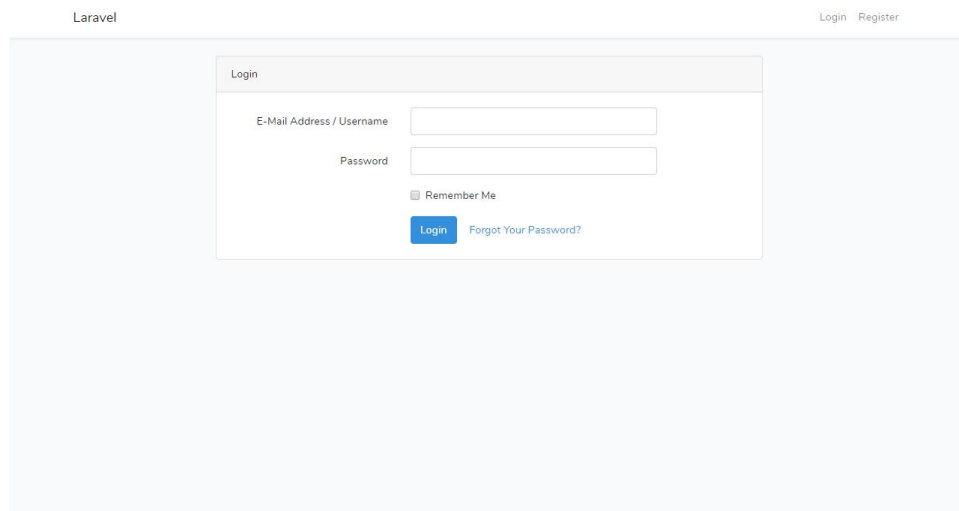
Gambar 4.1 Login Web
