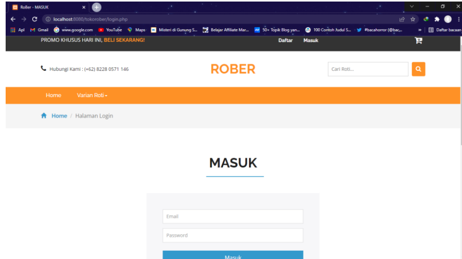
Gambar 4.7 Tampilan Login
