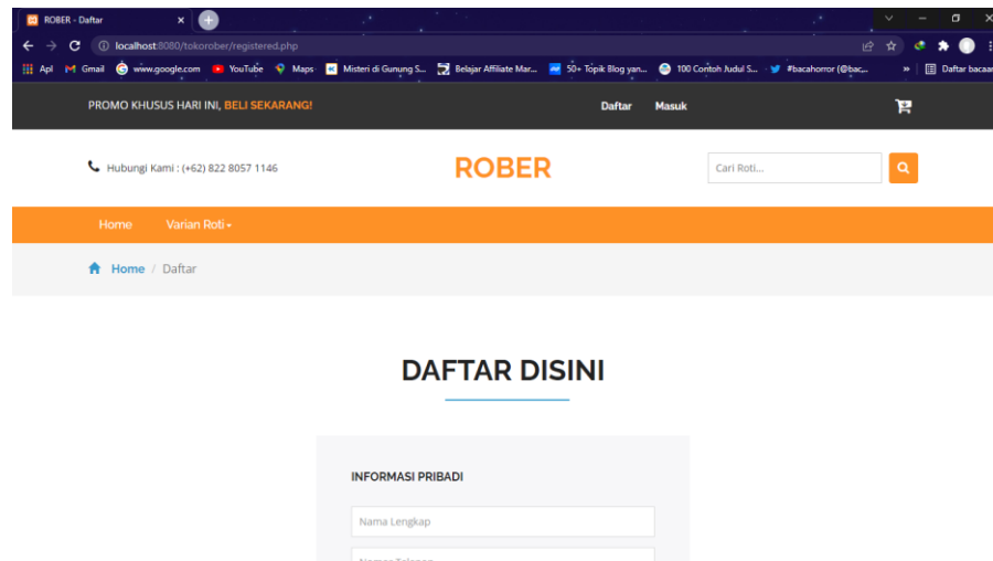
Gambar 4.8 Tampilan Daftar
