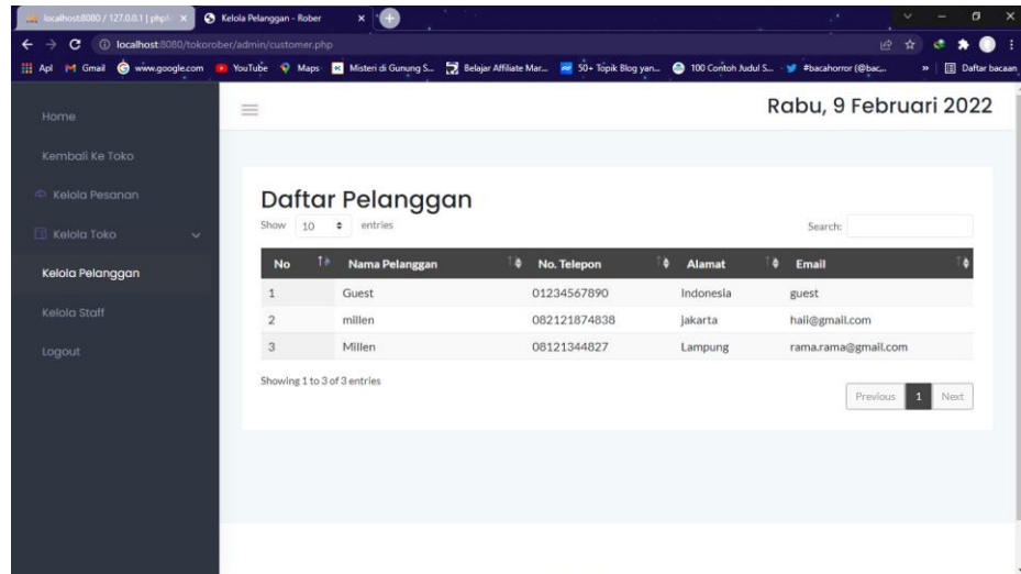
Gambar 4.10 Tampilan Pelanggan
