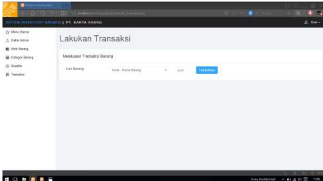
Gambar 3.25 Lakukan Transaksi
