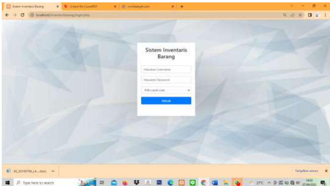
Gambar 3.9 Halaman Login
