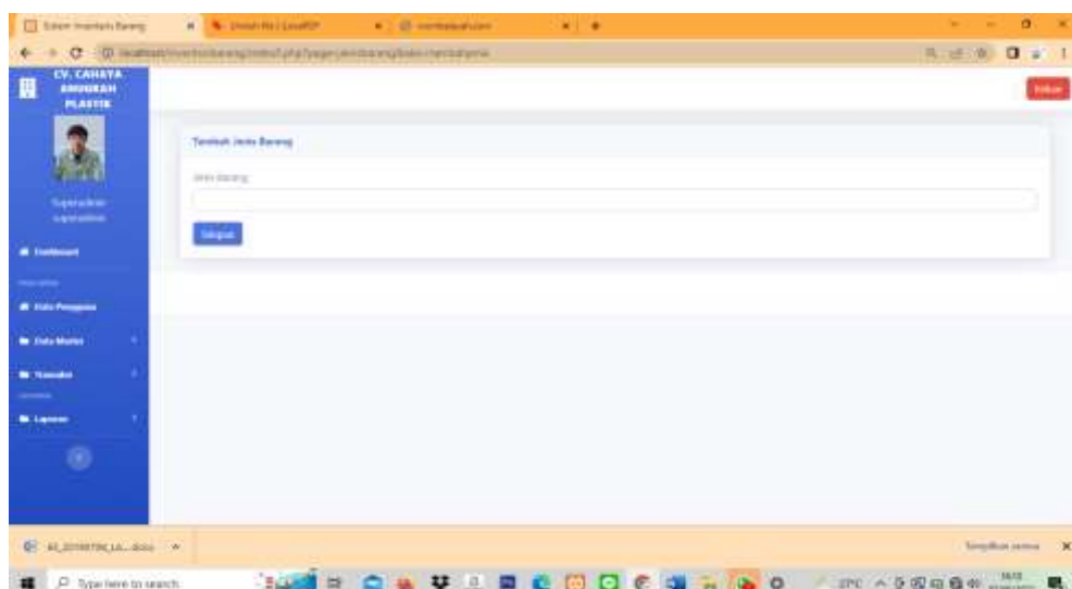
Gambar 3.19 Tambah Kategori
