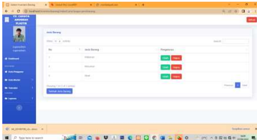
Gambar 3.18 Tampilan Kategori
