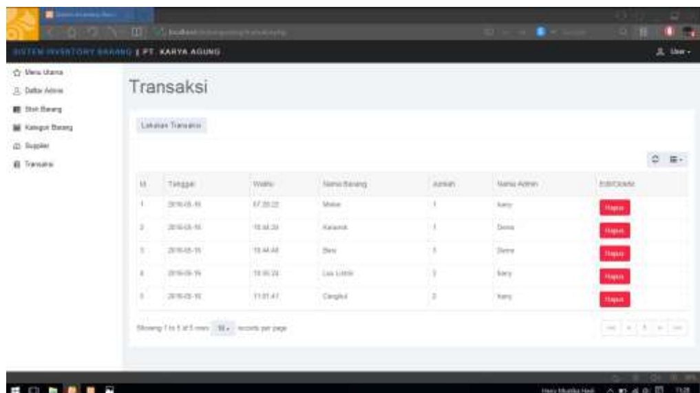
Gambar 3.24 Tampilan Transaksi
