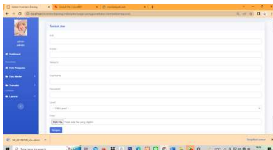
Gambar 3.13 Tambah Admin
