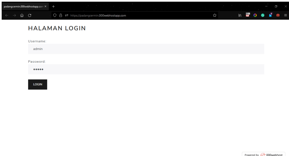
Gambar 4.1 Halaman login
