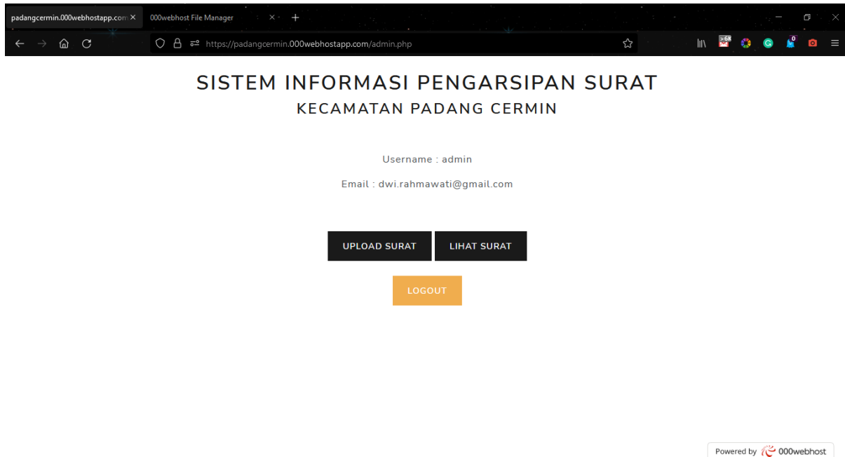
Gambar 4.2 Halaman utama
